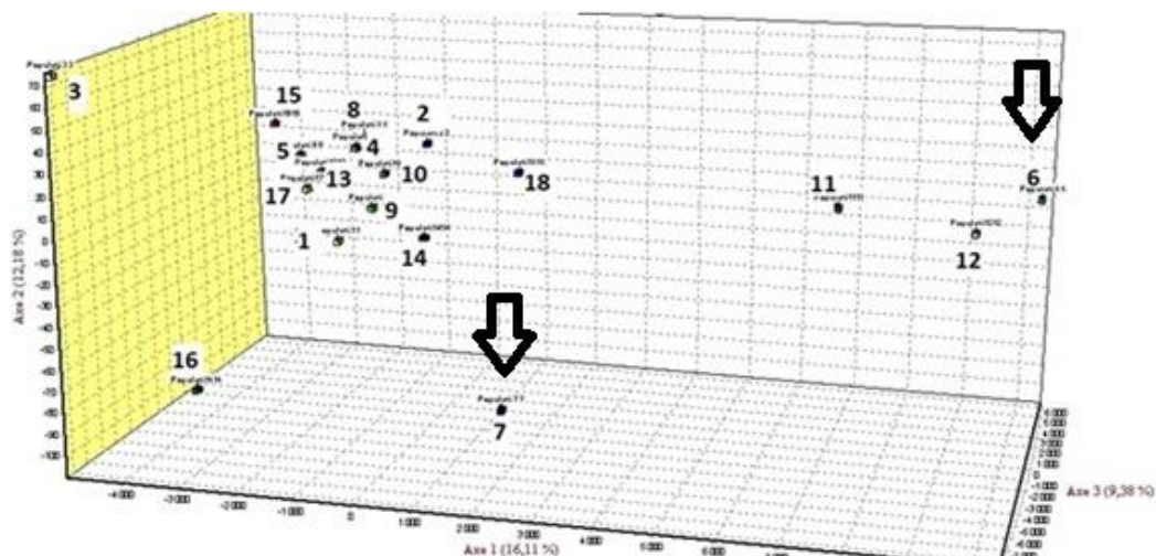
Obr. 3. Analýza hlavních komponent 3D PCA (Principal Component Analysis) zobrazuje středy 18 chovných populací pstruha duhového. Šipkou vyznačeny populace z Dánska (č. 6) a Irsko (č. 7).
